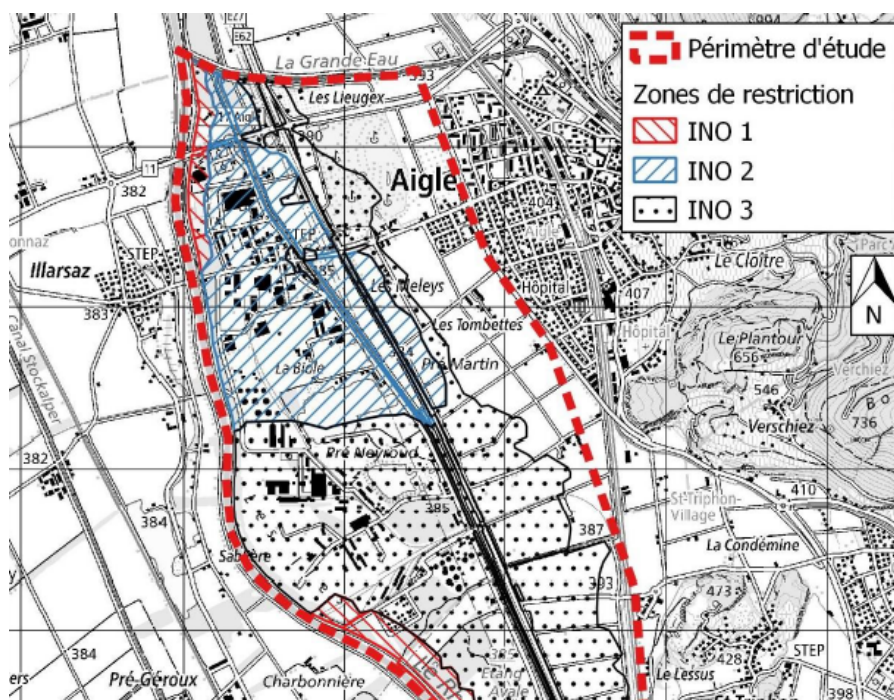
Figure 10 : Localisation des secteurs de restrictions liés aux dangers d'inondation du Rhône – Stucky
