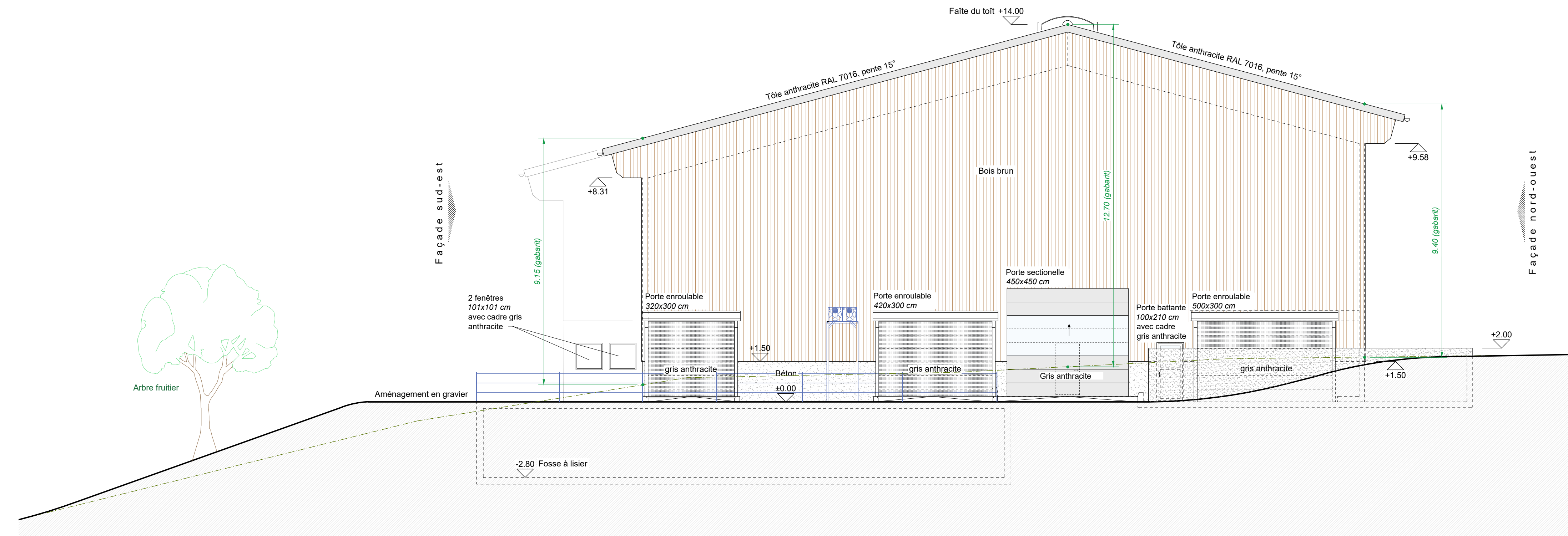
Façade nord-est
