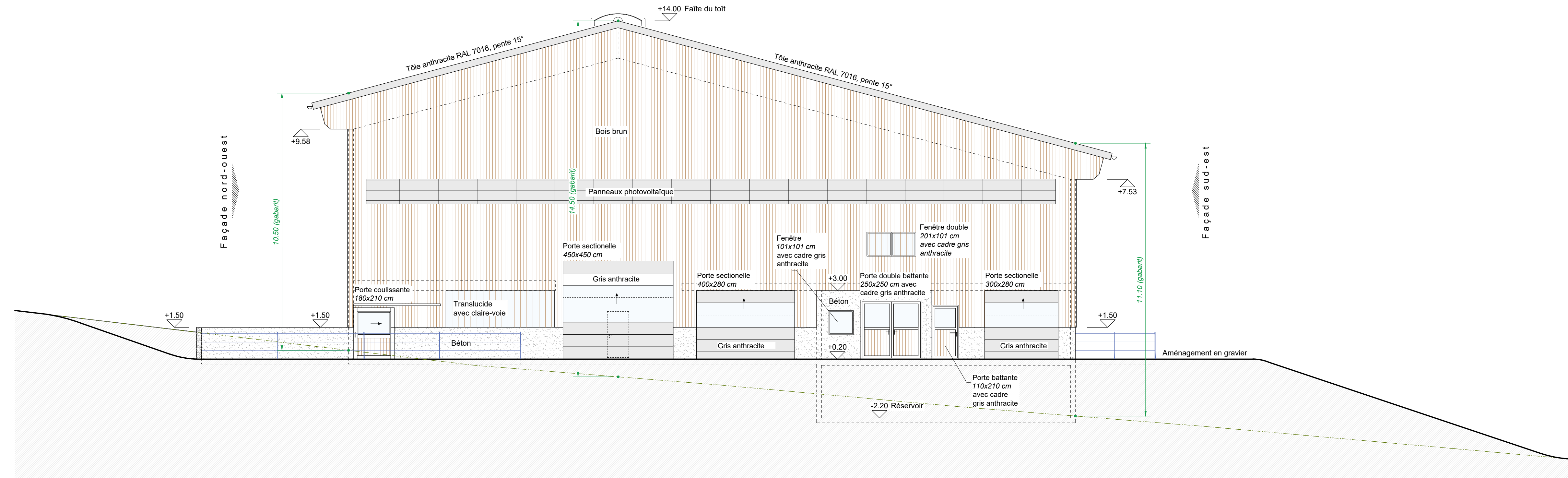
Façade sud-ouest
