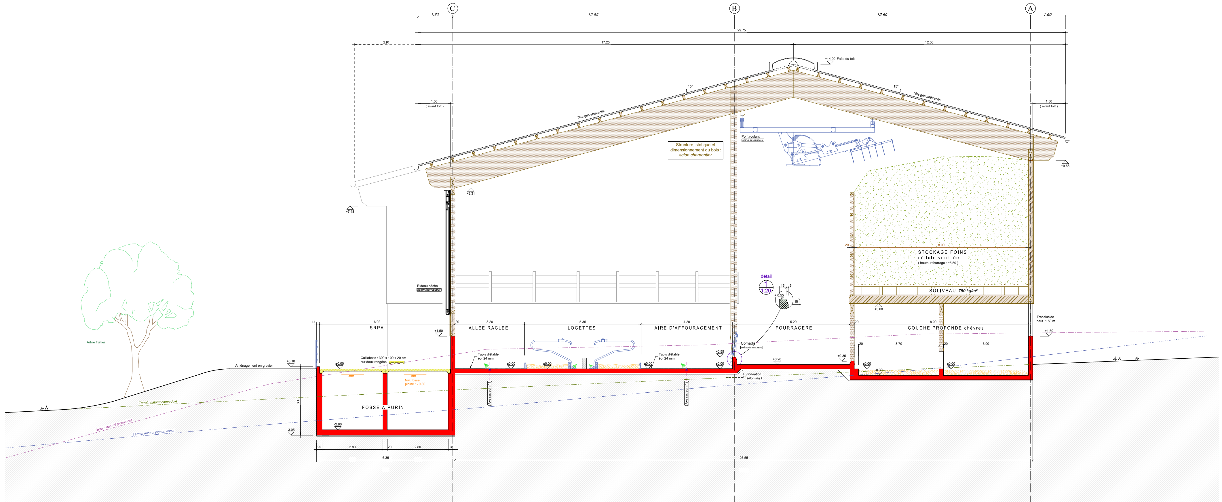
Coupe A-A
