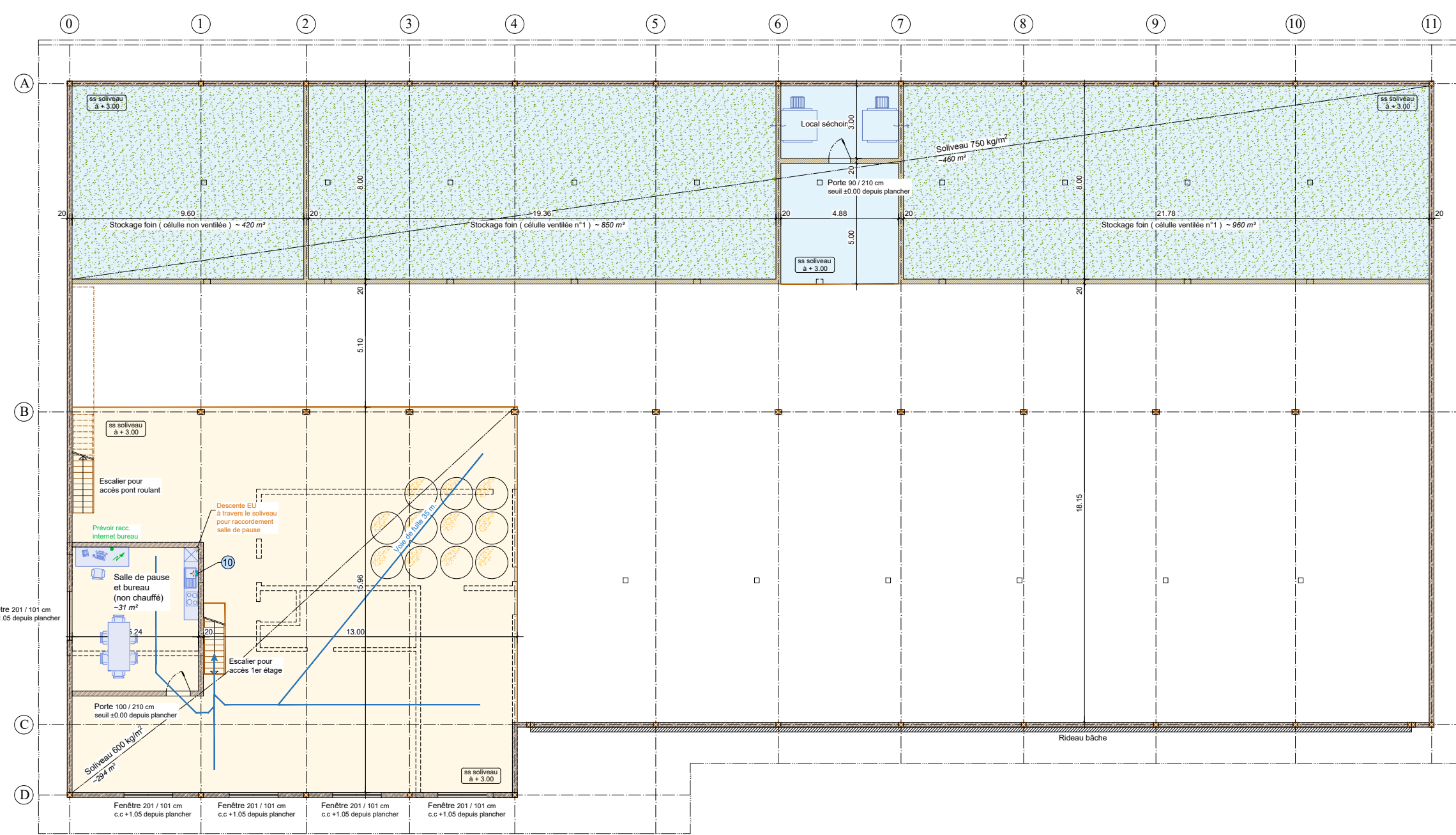
Vue Etage 1:200
